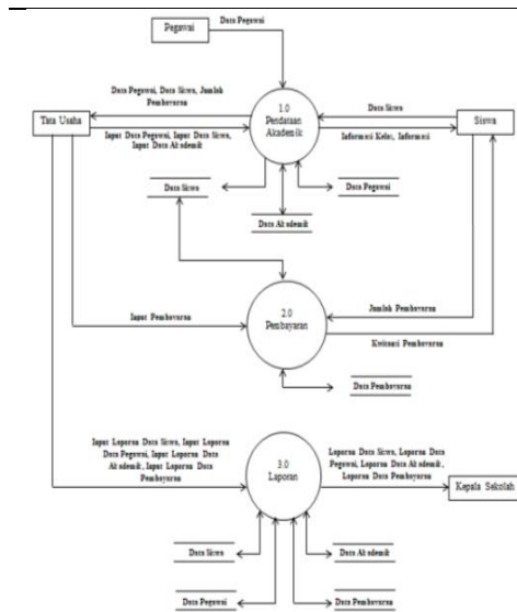
Gambar 3. Diagram Nol sistem administrasi dan akademik
