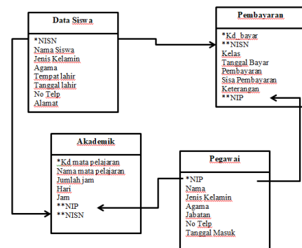
Gambar 4. Normalisasi
