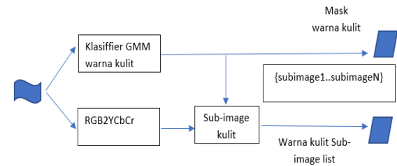
Gambar 2. Generasi Fitur Warna Kulit
